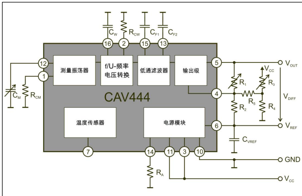
图 3: 零点和满度输出电压可调的完整电路图 CAV444
