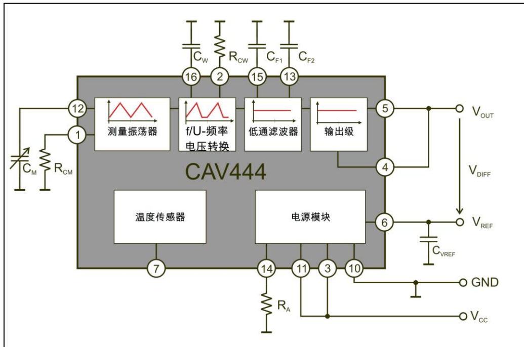
图 1: CAV444 的外接电路和信号测量转换过程
