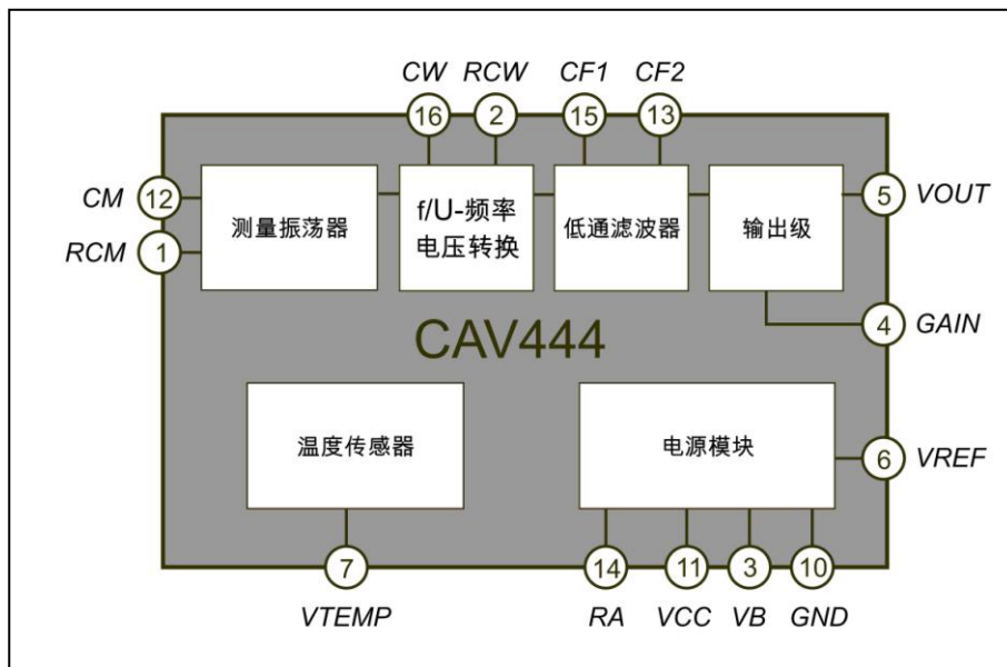
图 1：CAV444 电路方框图
