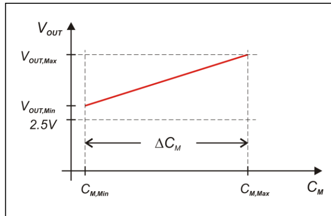
图 2: 输出电压 V_{OUT} (对地) 与测量电容 C_M 的关系曲线
