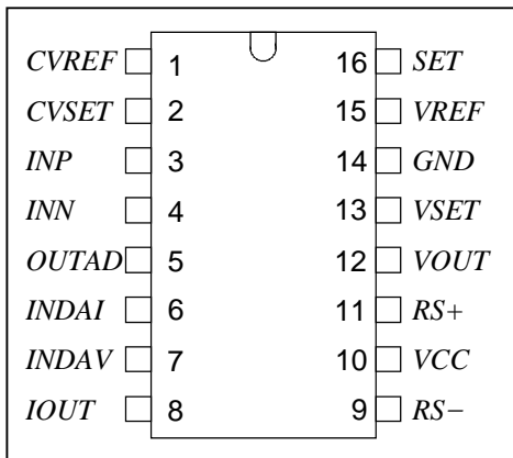
图 10: 管脚示意图
