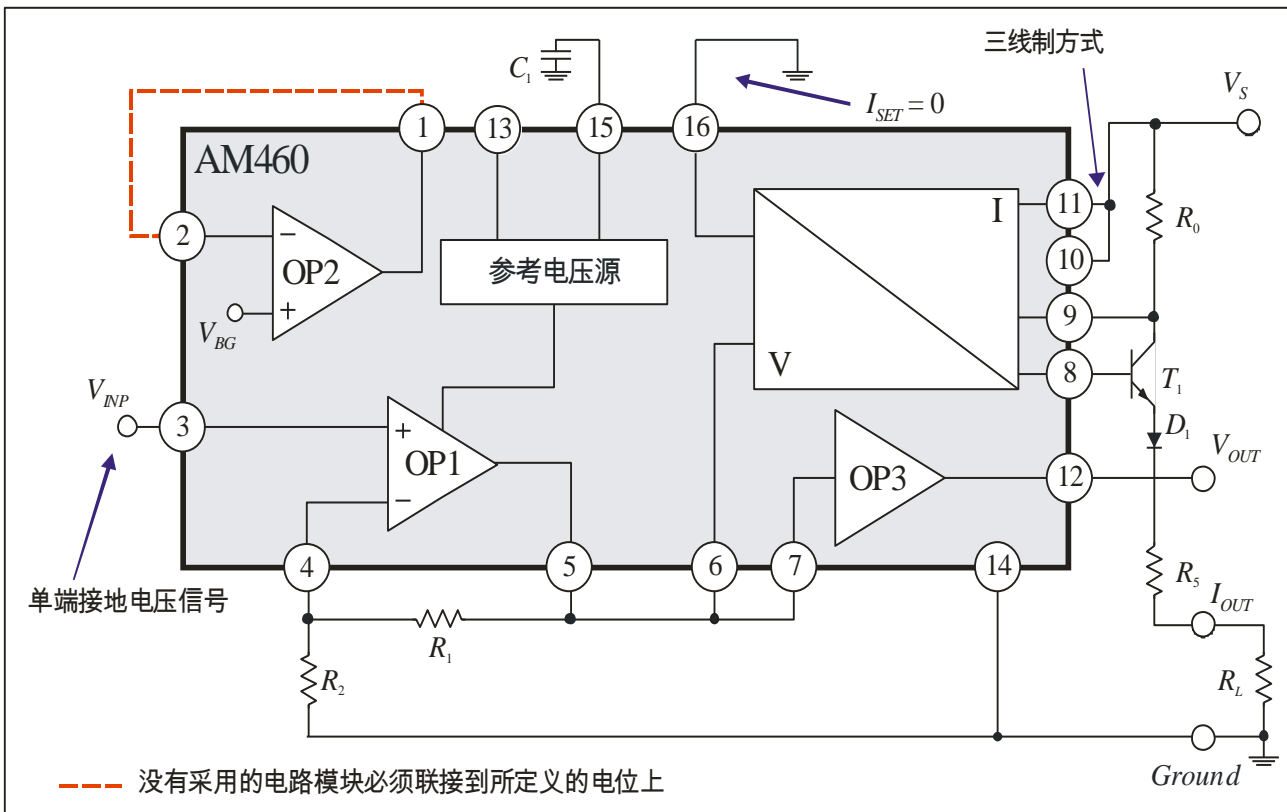
图 7：典型的电压电流平行输出应用电路
